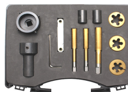
BGS1988 Wielmoer schroefdraad reparatie set. Réparation de filets de goujons de roues M12x1,25-12x1,5- 14x1,5
