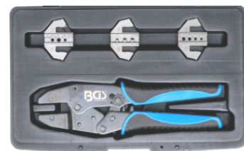
BGS70003 Krimptangen-set voor solar-steekverbindingen. Pince à sertir pour connecteurs solaires MC3/MC4/Tyco
