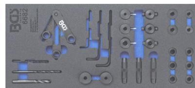
BGS6682 Cilinderkop-boormal gereedschapssset voor gebroken bouten. Op uit & inlaatspruitstukken, cilinderkoppen, versnellingsbakken, differentiëlen, motoren, etc. Extracteur de goujons cassés. M8 et M10 Pour collecteurs, culasses, différentiels, etc..
