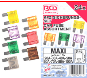
BGS8127 24 St./Pcs Maxi Zekeringen - fusibles 20 --> 100A 14,4 €
