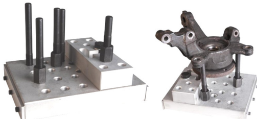
40017-WW Universele houder voor persen. 20T . Support universel presse.
