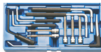
BGS8147 Demontageset voor airbags VW - Audi - BMW - Opel - Mercedes-Renault-Seat-Skoda,... Set de démontage pour airbags
