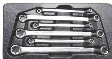
BGS2281 Stel 6 TXE ringsleutels. Jeu de 6 clés coudées TXE E6xE8, E7xE11, E10xE12, E14xE18, E16xE22, E20xE24 93 €
