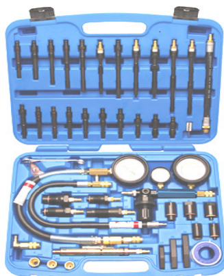
BGS8401 MASTER SET Compressiemeter en drukverlies tester benzine & diesel. Compressiomètre et testeur de fuites de cylindres diesel et essence
