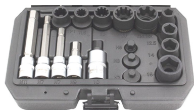
3357-WW Master set doppen voor remmen. Douilles pour freins. Allen 7-8-9-11mm. 5 kant/pans 10mm. 7 kant/pans 22 - 10 kant/pans 10-11,5-12,5- 14-15-19-20mm
