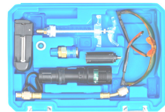
K8725 Airco UV lekzoeklamp oplaadbaar met brillen. Lampe UV rechargeable pour la détection de fuites Airco avec lunettes.
