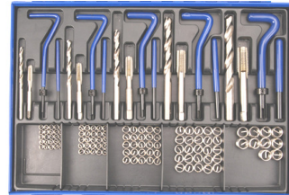
51001-WW Schroefdraad reparatieset. M5-6-8-10-12 Jeu de réparation de 92 €
