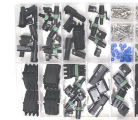
BGS9096 232 St./Pcs Type Delphi® Conecteurs waterproof connectors 114 €
