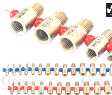
Snel draadkaliber binnen en buiten. Jauge rapide intérieure/extérieure 5684P M4-M5-M6-M7-M8x1,0-M8x1,25- M10x1,0-M10x1,25-M10x1,5-M12x1,25- M12x1,5-M12x1,75 18 € 5685P Metric & duim / pouces UNF & UNC --> 1/2" & M4-M12 30 €
