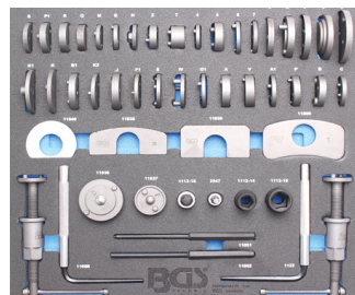
BGS1102 50 ST. / PCS. Terugstelset remzadelzuigers links-rechts 50-dlg. Set d'outils repousse piston de freins gauche-droite 50pcs 199 €
