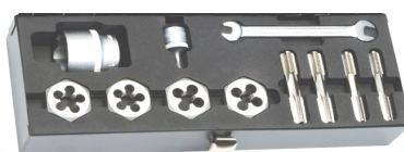
VOL48647 Wielmoer schroefdraad reparatie set. Réparation de filets de goujons de roues M12x1,25-12x1,5-14x1,25-14x1,5
