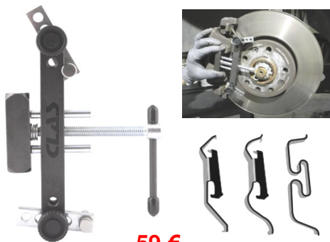
OM2121 Trekker voor remklauwen veer. Extracteur de ressort d'étrier de freins. Tijdsbesparing en veiliger. Gain de temps et de sécurité. Universal
