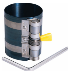
Zuigveer spanband. Collier à segments
